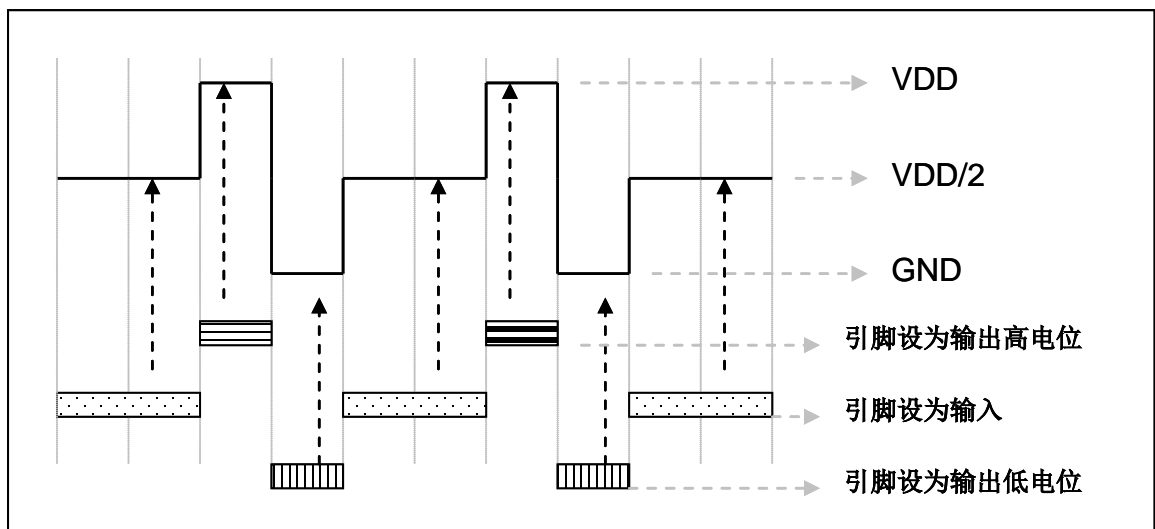
图 8: 使用半电位偏置电压
